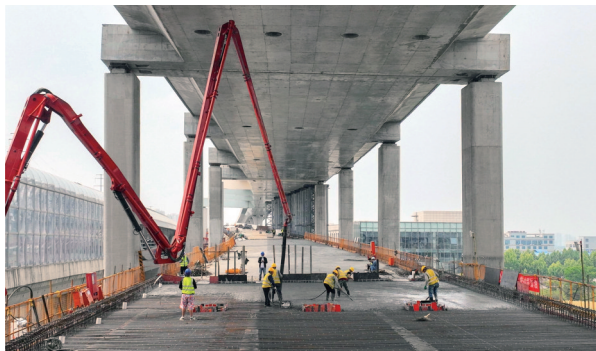
▲混凝土浇筑
