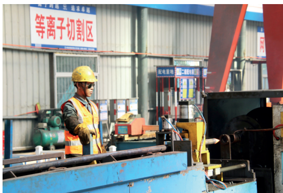
▲隧道锚杆自动化加工
