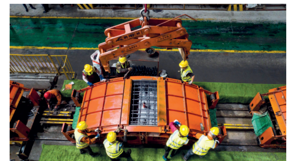
城轨分公司安徽智能制造公司作业人员对管模具加固密封 杨锋 摄
