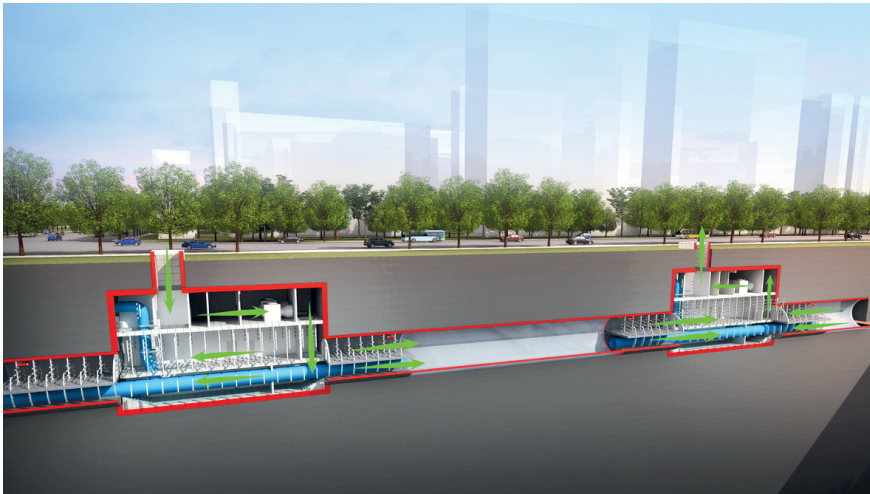
工作井及区间剖面图
