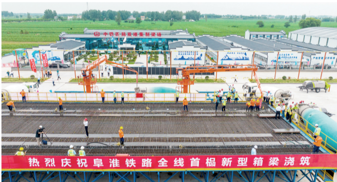
阜淮铁路全线首榀新型箱梁浇筑准备就绪
