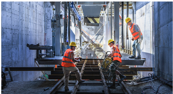
盾构机台车下井准备进入站台
