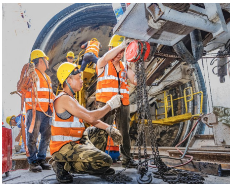
工人进行盾构机螺机安装
