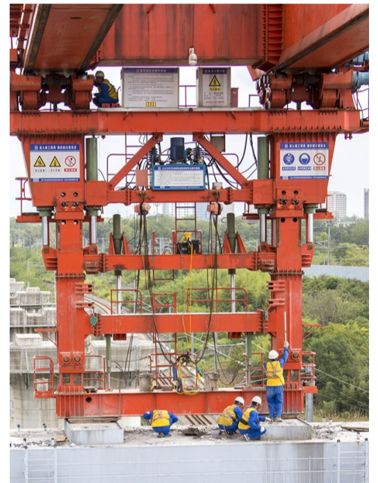
昌景黄铁路跨京台高速公路特大桥梁架设施
