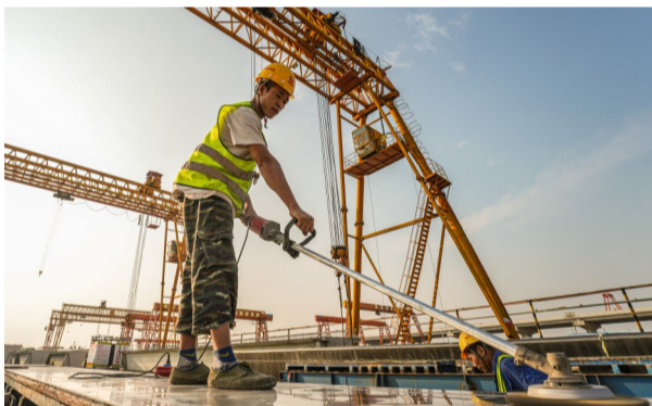
工人对预制梁内模进行打磨
