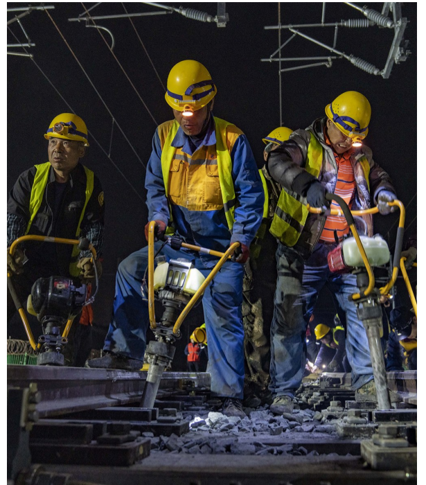
工人正在使用机械对道砟进行高频振动捣固
