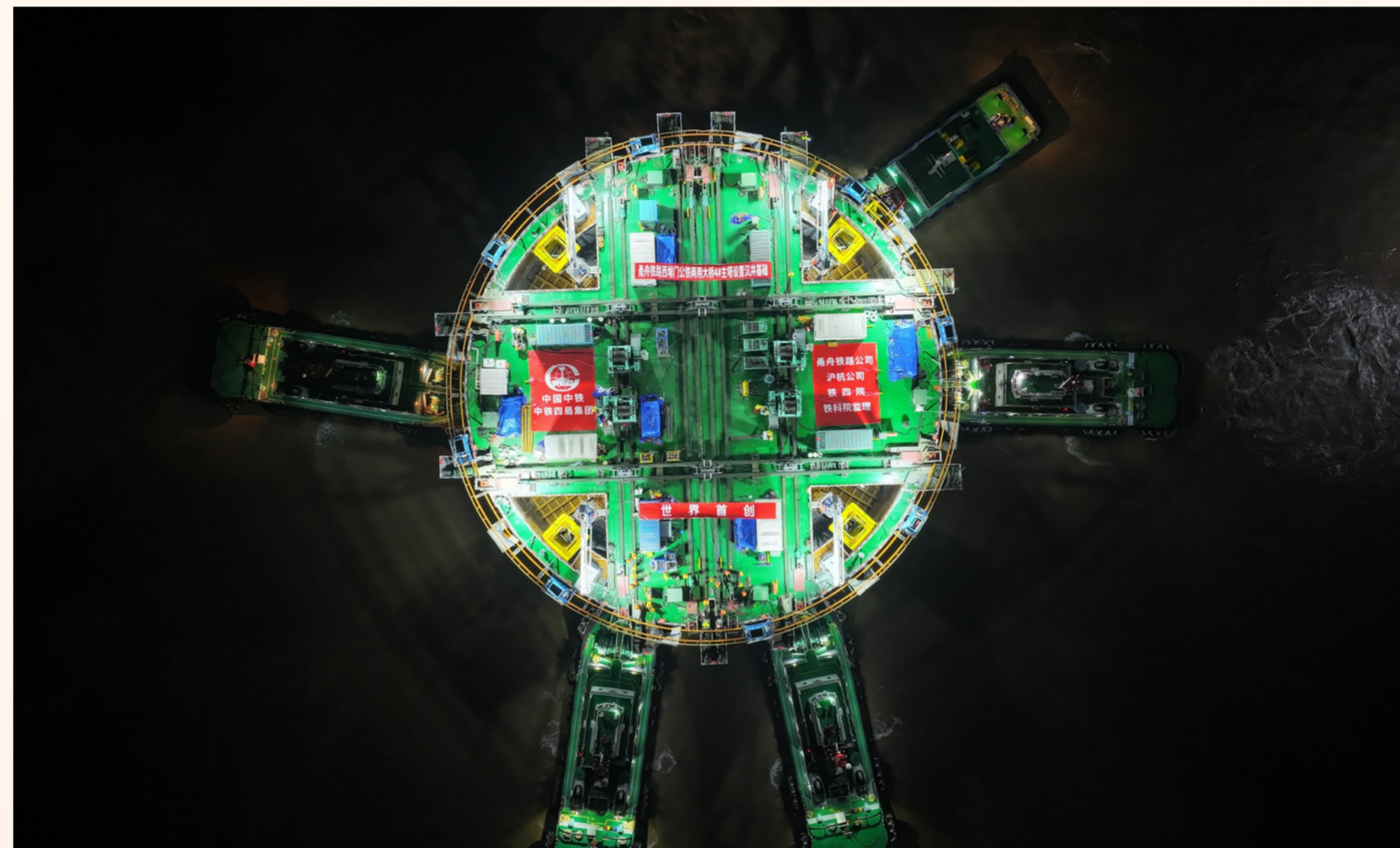
甬(宁波)舟(山)铁路西堠门公铁两用大桥项目4号墩主塔设置钢沉井过缆施工
