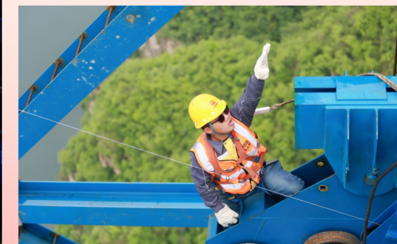
一公司济(源)新(安)黄河大桥项目先导索架设施工现场,建设者正在指挥卷扬机收缆 陶冶 摄
