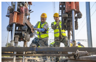
工人正在进行线路捣固作业
