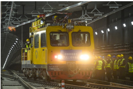
工作人员对接触网冷滑车相关参数和数据采集系统做最后的确认
