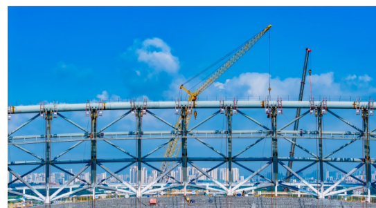
体育场索结构安装
